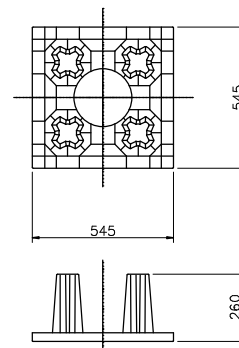
SSBB本体詳細図 S=1:20(10)
